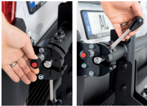
Einfach und gefahrlos entriegeln und schwenken
